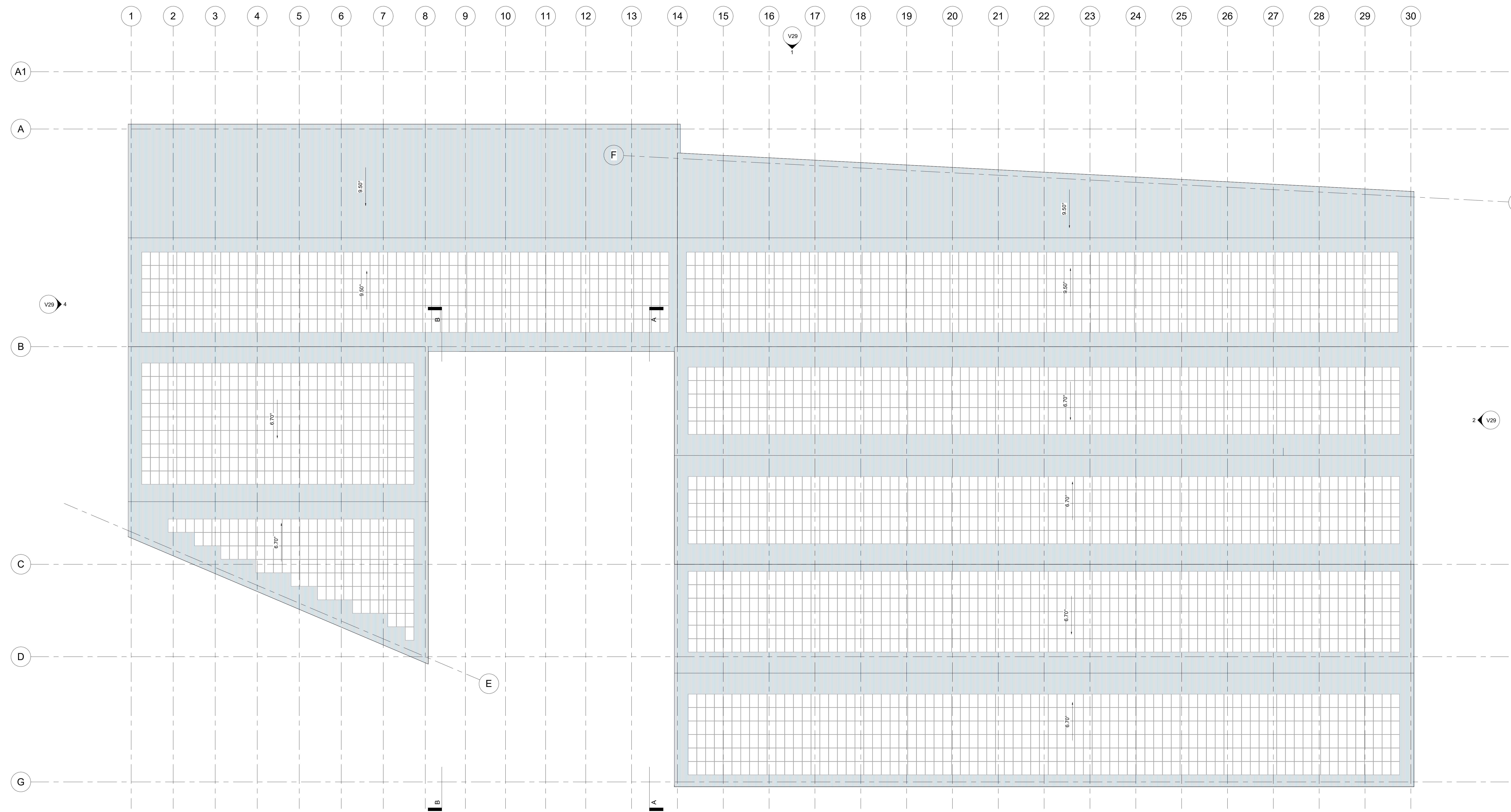
3 V29 EAVES LAYOUT Scale 1 : 200
